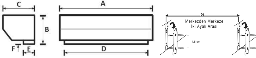
GENEL TİP SU VE BUHAR SERPANTİNLİ HAVA PERDELERİ EBAT VE AĞIRLIK TABLOSU
